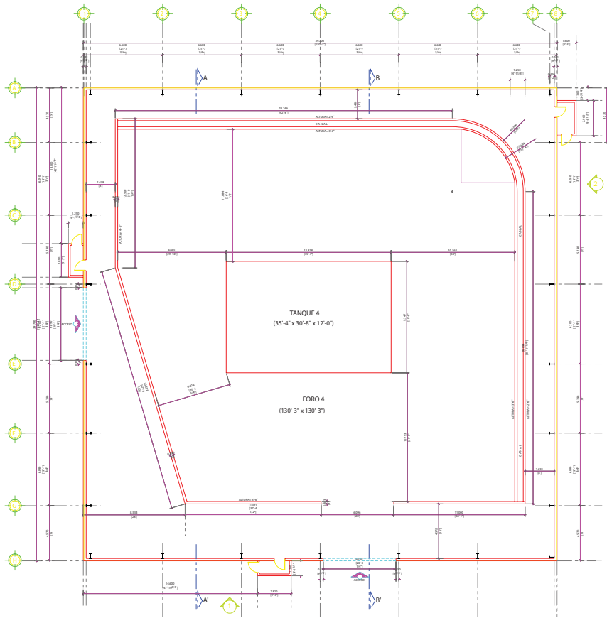
PLANTA ARQUITECTONICA FORO 4
