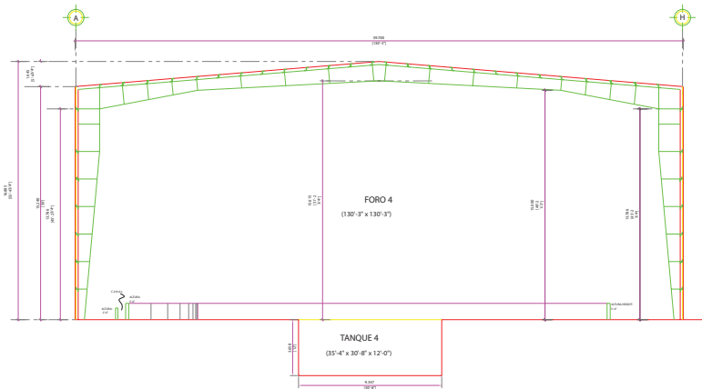
CORTE B-B' - FORO 4
