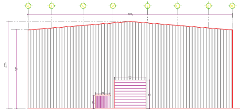
2 FACHADA NORTE - FORO 4
